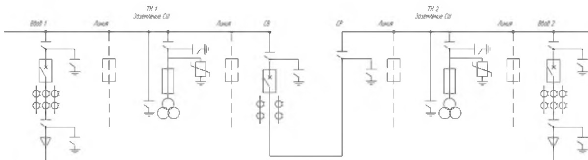
Рисунок 2 - Рекомендуемая схема организации главных цепей (однорядное исполнение)
