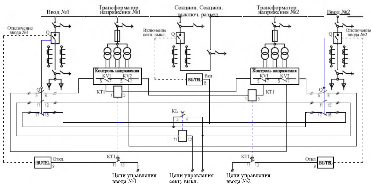
Рисунок 15 - Цепи АВР
