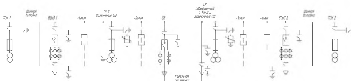
Рисунок 3 - Рекомендуемая схема организации главных цепей (двухрядное исполнение, стыковка между рядами шинным мостом по сборным шинам)
