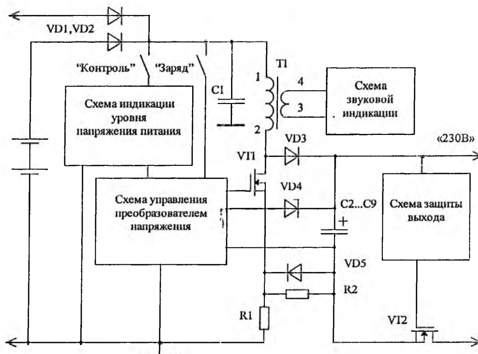
Рисунок Г.1 - Блок автономного включения BAV/TEL-220-02
