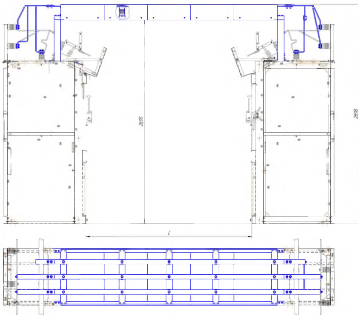
Рисунок 13 - Шинный мост
