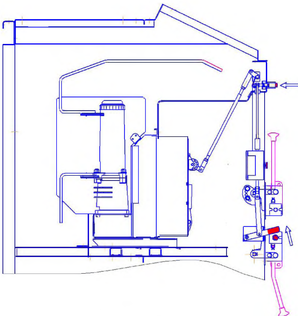
Рисунок 11 – Выключатель отключен
