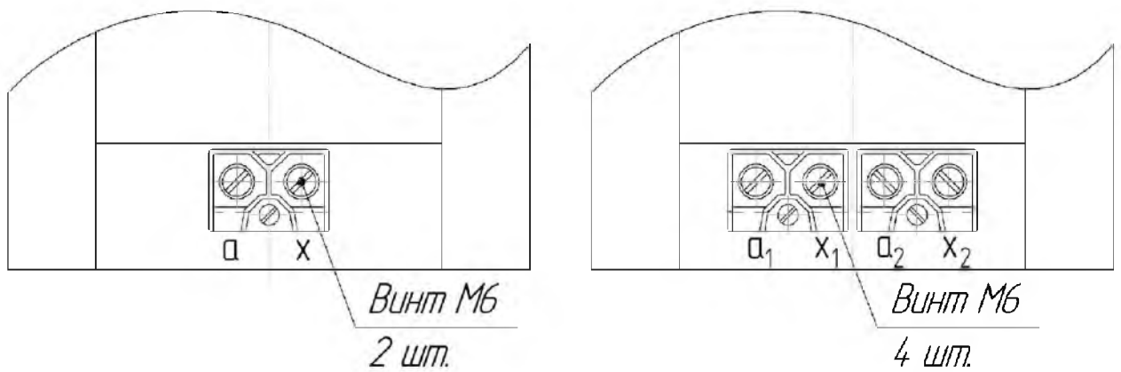
Рисунок 6 - Расположение вторичных выводов трансформаторов НОЛ-СЭЦ-6-20 и НОЛ-СЭЦ-10-20
