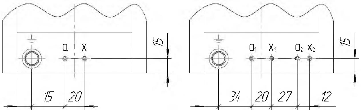
Рисунок 7 - Расположение вторичных выводов трансформаторов НОЛ-СЭЦ-6-40 и НОЛ-СЭЦ-10-40
