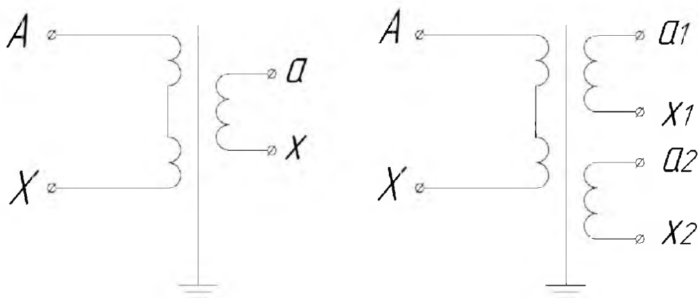
Рисунок 4 - Принципиальные электрические схемы трансформаторов НОЛ-СЭЦ
