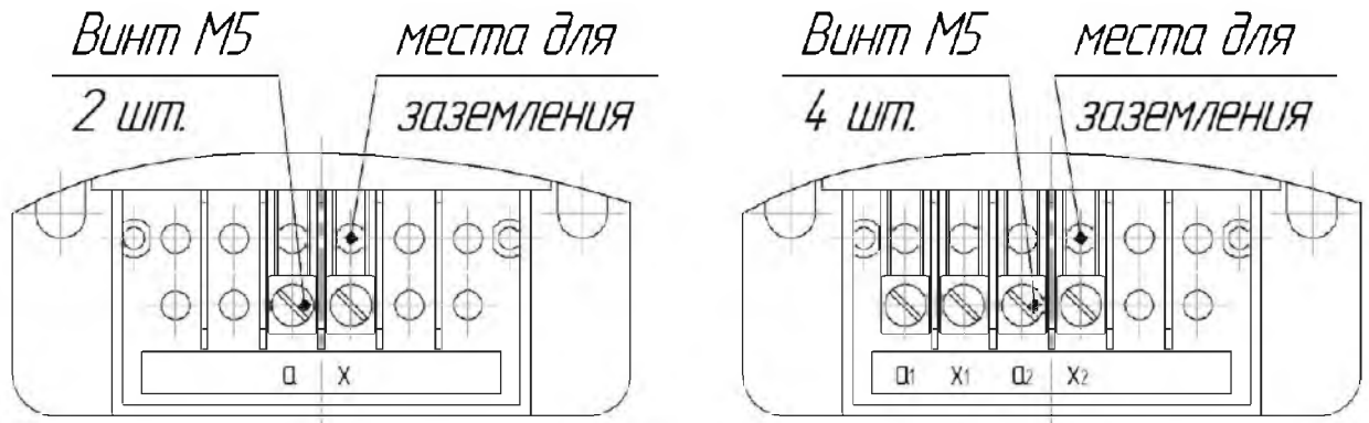
Рисунок 5 - Расположение вторичных выводов трансформаторов НОЛ-СЭЦ-6 и НОЛ-СЭЦ-10
