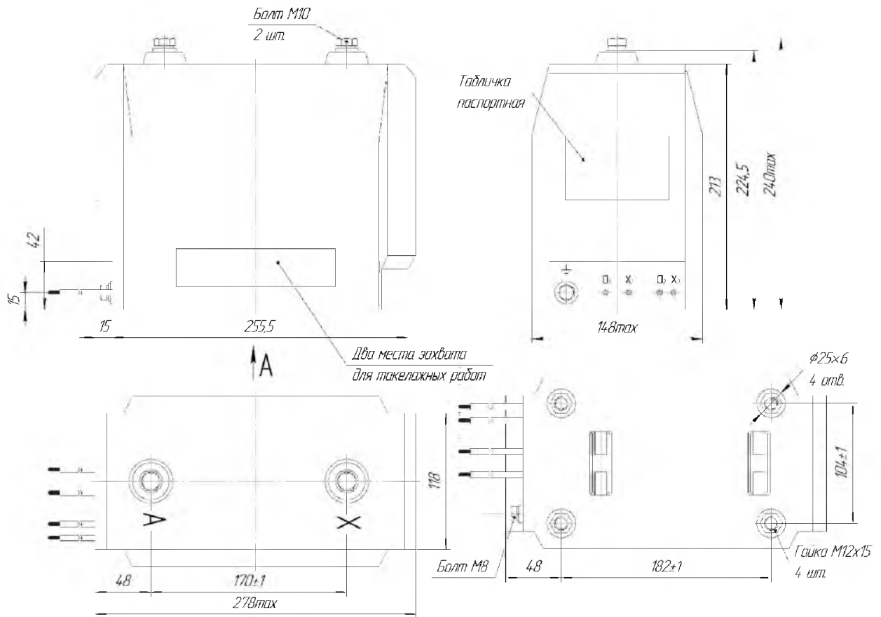
Рисунок 3 - Габаритные, установочные и присоединительные размеры трансформаторов напряжения НОЛ-СЭЦ-6-40 и НОЛ-СЭЦ-10-40
