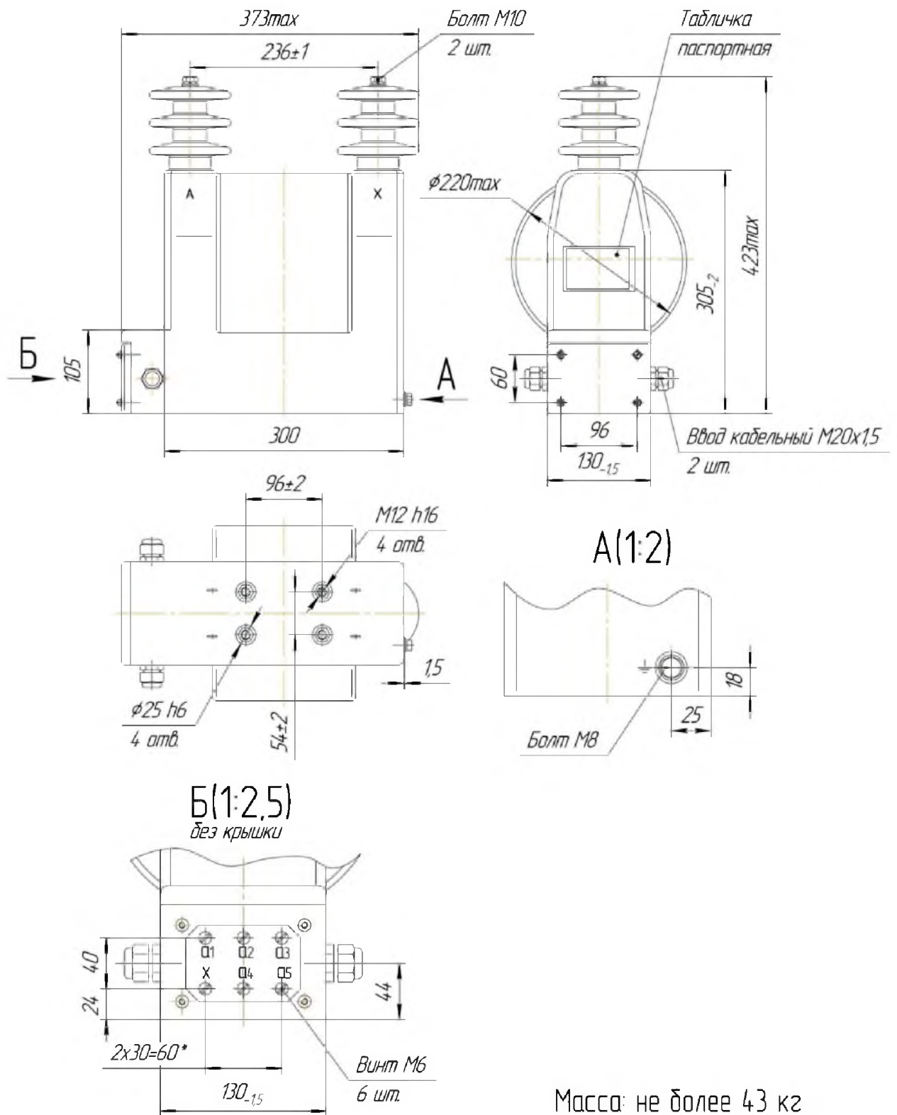
Рисунок 1 - Габаритные, установочные и присоединительные размеры трансформатора ОЛС-СЭЦ-0,63(1,25)/6(10)
