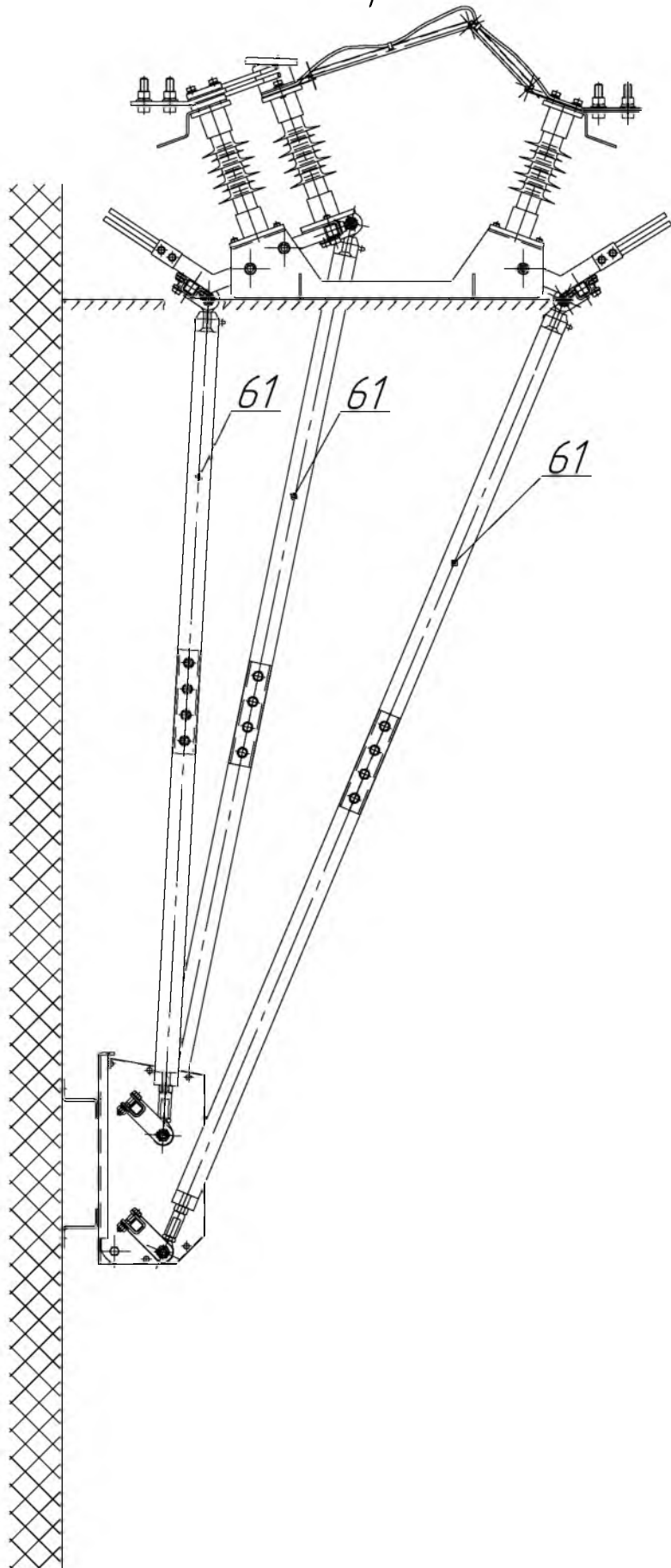
Рисунок Е.1 Пример установки разъединителя 61-соединительная тяга (тяги 51, 52 и труба 25x3,2 ГОСТ 3263).
