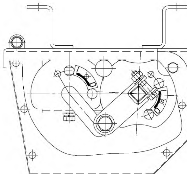
Рисунок Г.1. Привод ПР СЭЦ-01 УХЛ1
