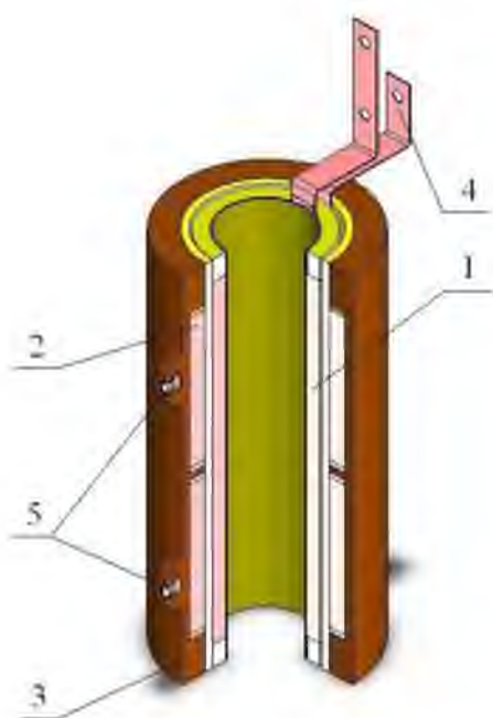
Рисунок 3а - Обмотки НН и ВН. (без регулирования ПБВ).
