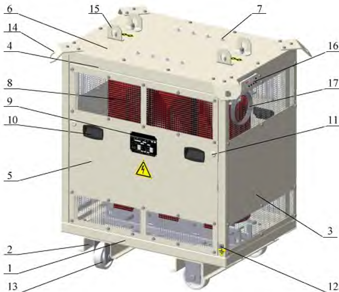
Рисунок 8 - Конструкция трансформатора типа ТЛСЗ-СЭЩ (исполнения -02, -03, -05).
