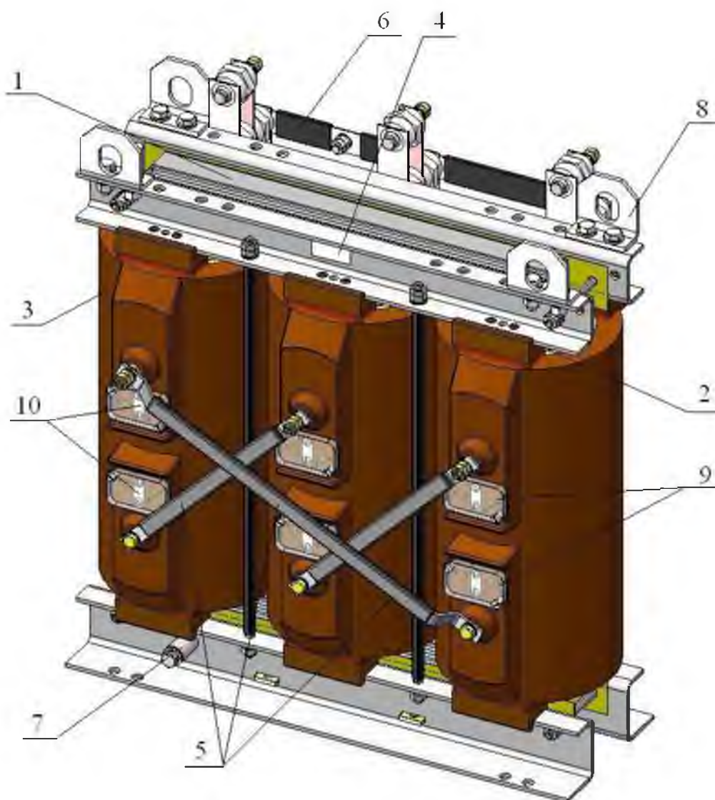
Рисунок 5 - Конструкция трансформатора типа ТЛС-СЭЦ (исполнения -01, -03).
