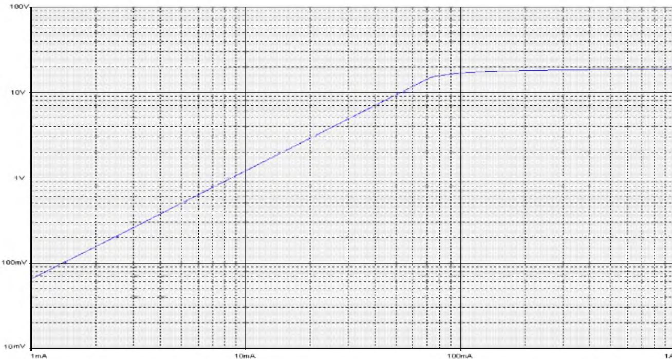
ВАХ вторичной обмотки для измерения с КТ 0,5S, номинальной нагрузкой 10 В·А и K_{\text{Бном}} = 10 трансформаторов с первичными токами 400, 800 А. Сопrotивление обмотки постоянному току – 0,105 Ом.
