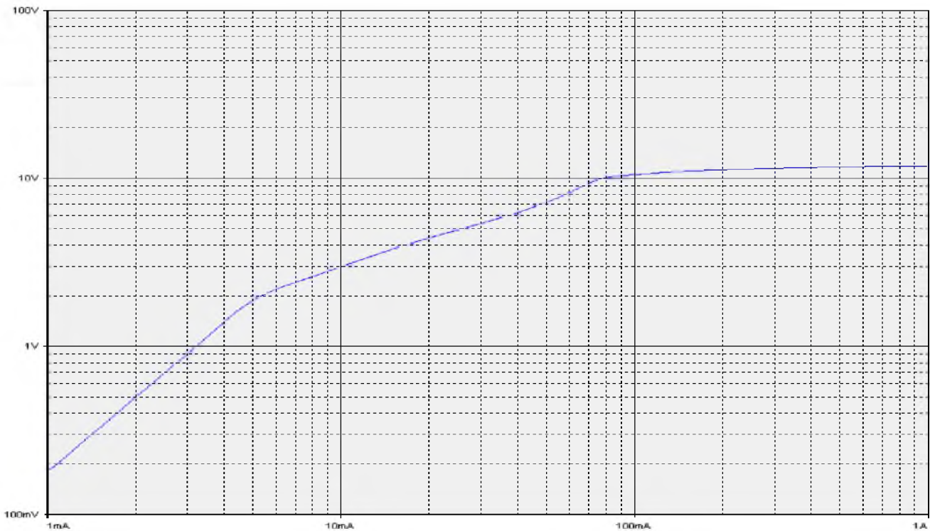
ВАХ вторичной обмотки для измерения с КТ 0,2; 0,2S, номинальной нагрузкой 10 В·А и K_{\text{БНОМ}}=10 трансформаторов с первичными токами 400, 800 А. Сопротивление обмотки постоянному току – 0,125 Ом.
