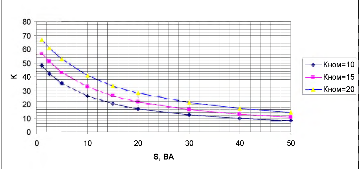
Кривые предельной кратности вторичных обмоток для защиты с классами точности 5Р и 10Р и номинальной нагрузкой 30 ВА трансформаторов с первичным током 2000А
