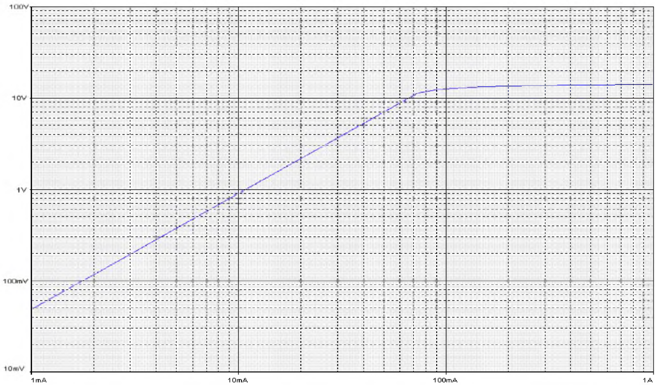
ВАХ вторичной обмотки для измерения с КТ 0,5, номинальной нагрузкой 10 В·А и K_{\text{Бном}} = 10 трансформаторов с первичными токами 400, 800 А. Сопrotивление обмотки постоянному току – 0,094 Ом.
