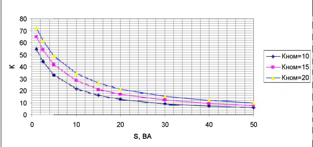
Кривые предельной кратности вторичных обмоток для защиты с классами точности 5Р и 10Р и номинальной нагрузкой 20 ВА трансформаторов с первичным током 1000А
