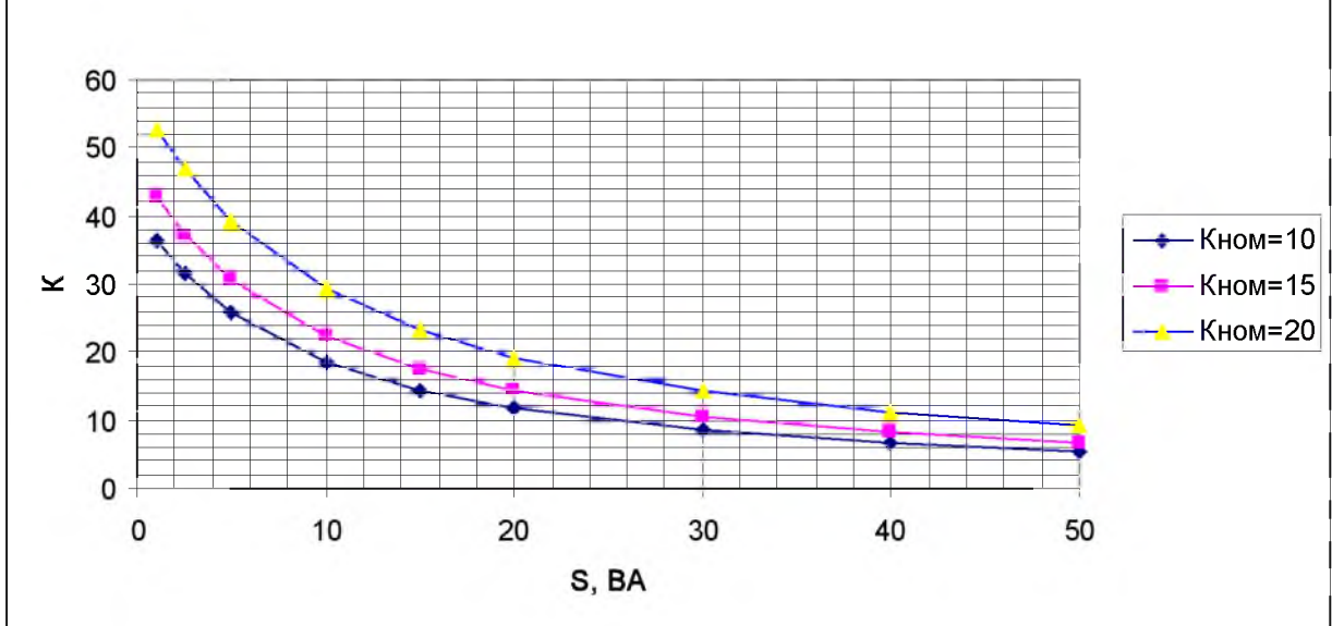
Кривые предельной кратности вторичных обмоток для защиты с классами точности 5P и 10P и номинальной нагрузкой 15 ВА трансформаторов с первичным током 2000А
