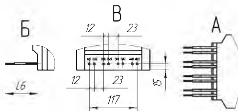
Рисунок 15 Остальное – см. рисунок 1
