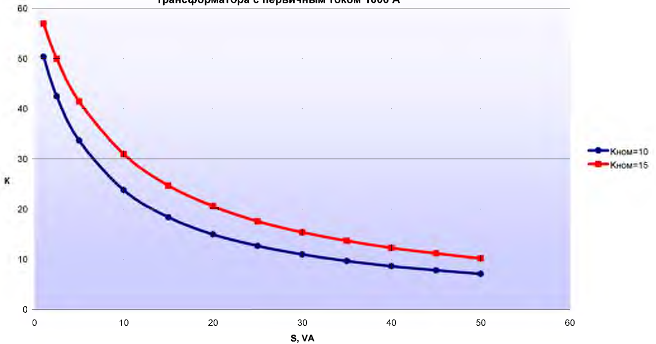
Кривая предельной кратности вторичной обмотки для защиты с классом точности 5Р, 10Р и номинальной нагрузкой 30 ВА трансформатора с первичным током 1000 А
