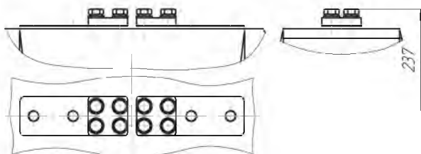
Рисунок 2 Остальное см. рисунок 1, 3, 4 Трансформатор тока с переключением на первичной стороне (максимальный ток 600А)
