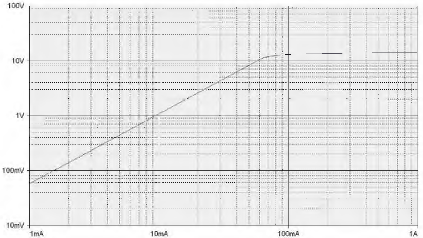
ВАХ вторичной обмотки для измерения с КТ 0,5, номинальной нагрузкой 10В·А и K_{\text{БНОМ}}=10 трансформаторов с первичными токами 400, 800 А. Сопротивление обмотки постоянному току – 0,10 Ом.
