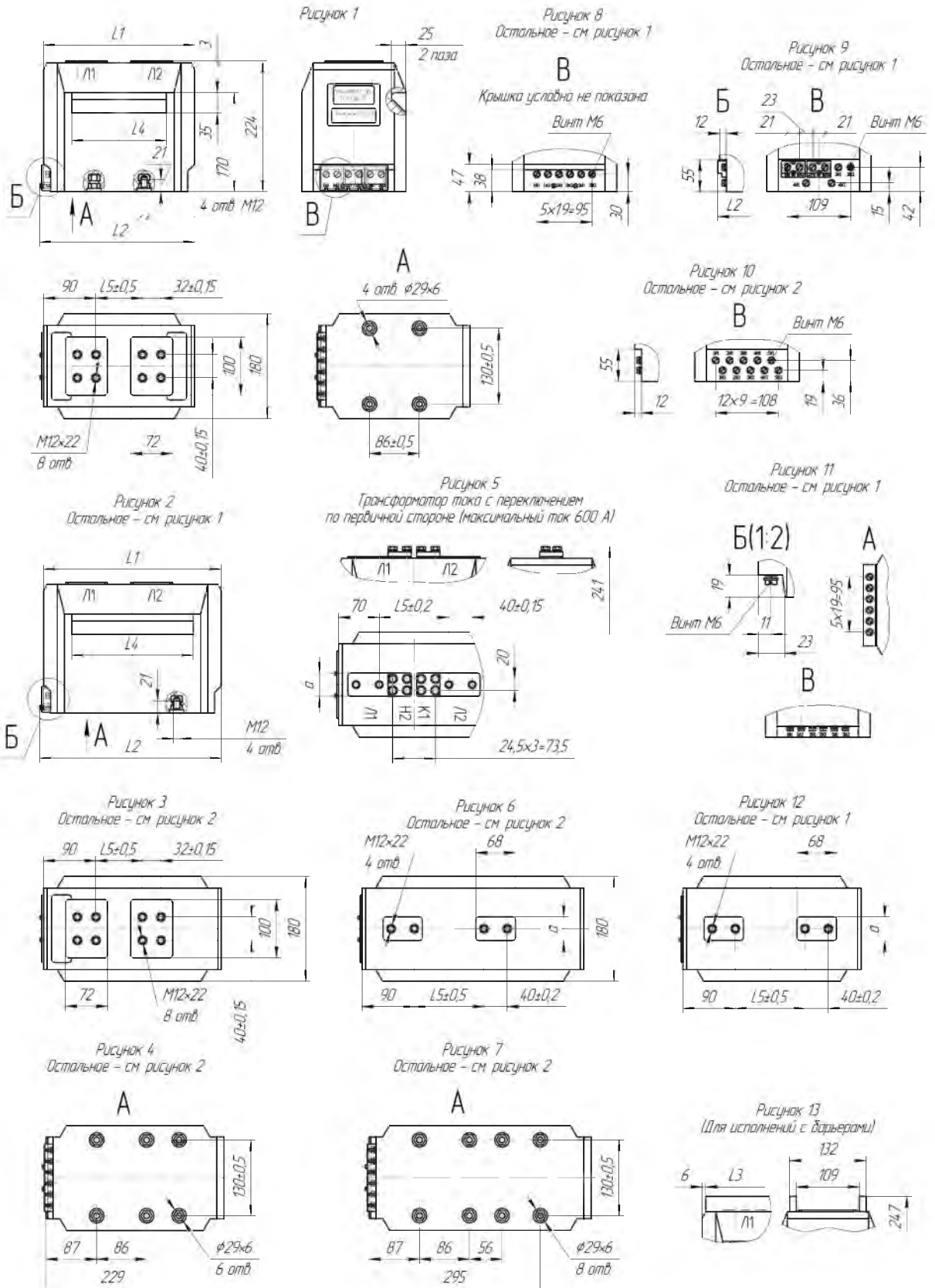
Габаритные, установочные, присоединительные размеры и масса трансформатора тока ТОЛ-СЭЩ-10 исполнений 11÷84-1
