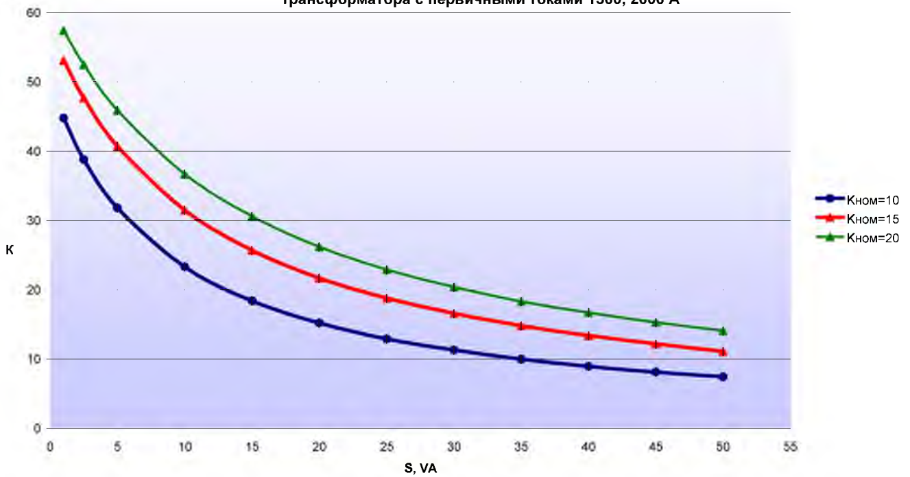
Кривая предельной кратности вторичной обмотки для защиты с классом точности 5Р, 10Р и номинальной нагрузкой 30 ВА трансформатора с первичными токами 1500, 2000 А
