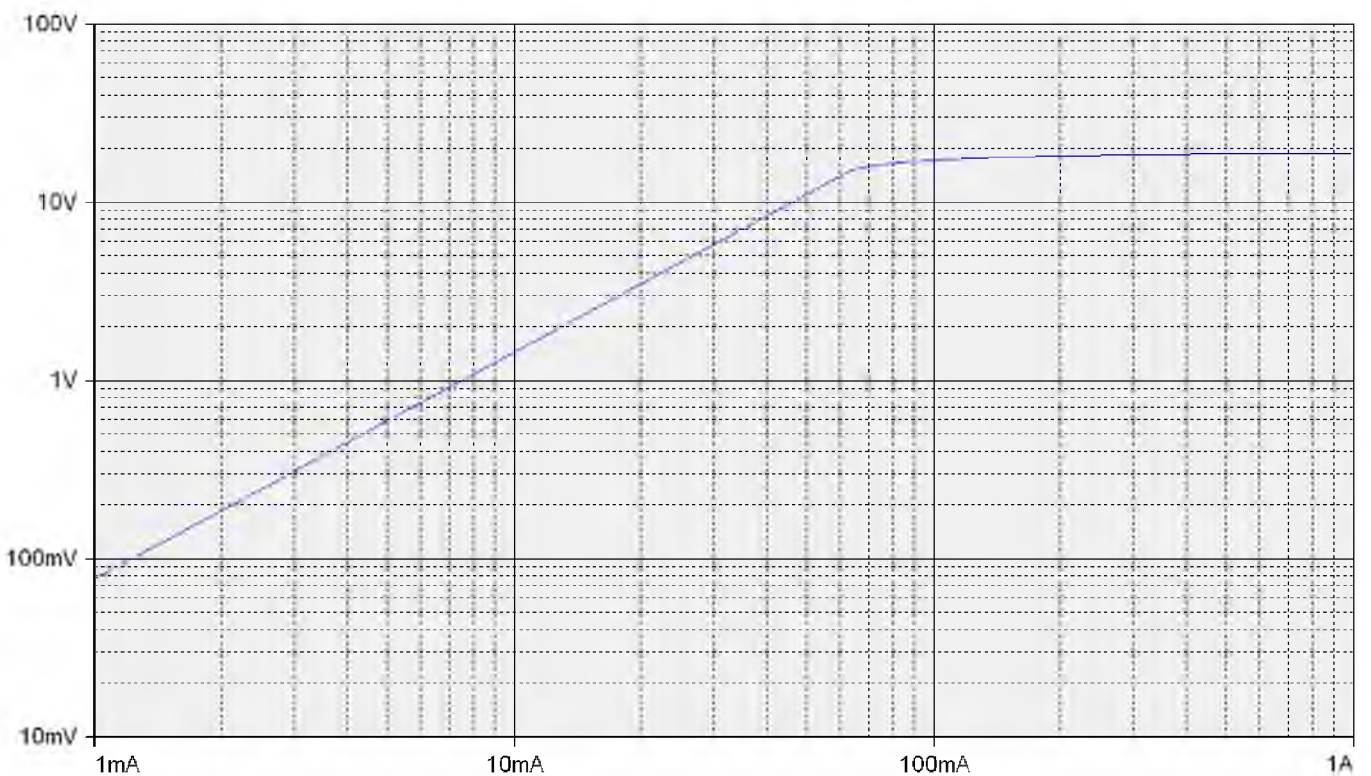
ВАХ вторичной обмотки для измерения с КТ 0,5S, номинальной нагрузкой 10В·А и K_{\text{БНОМ}}=10 трансформаторов с первичными токами 400, 800 А. Сопротивление обмотки постоянному току – 0,11 Ом.
