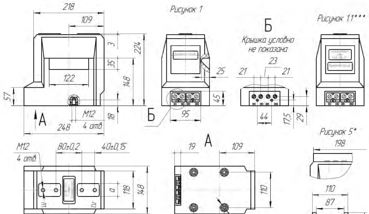
Рисунок 2 Остальное см. рисунок 1
