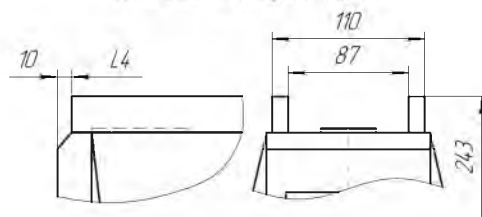
Рисунок 3 Трансформатор тока с барьерами Остальное см. рисунки 1, 2, 4
