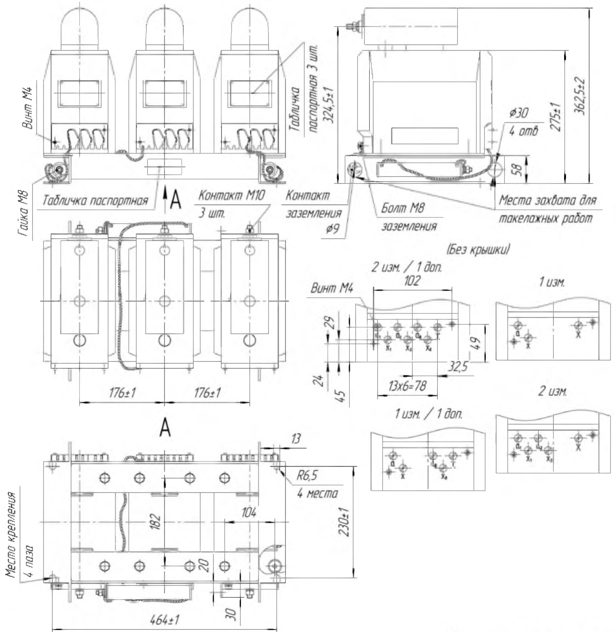
Рис.А.8 Габаритные, установочные и присоединительные размеры трехфазной группы измерительных трансформаторов 3 х ЗНОЛ – СЭЦ – 6(10) – 22
