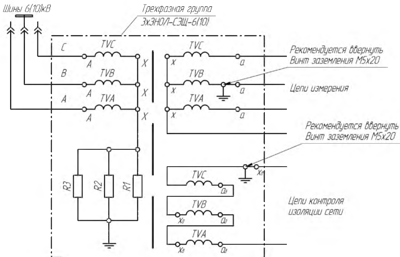
Рис.Б.1 Принципиальная электрическая схема соединения обмоток трехфазной группы измерительных трансформаторов 3 x ЗНОЛ – СЭЩ – 6(10)
