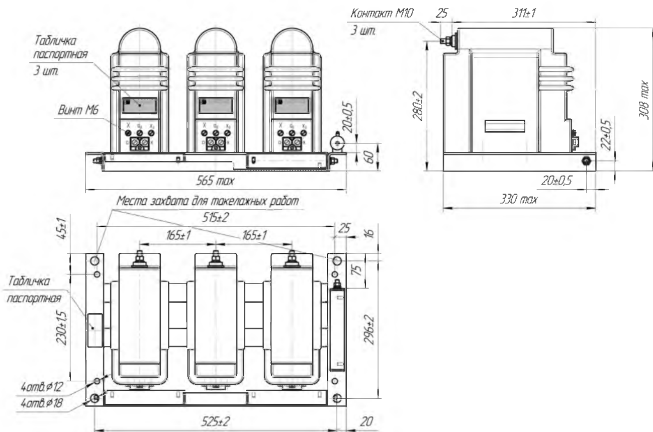
Рис.А.12 Габаритные, установочные и присоединительные размеры трехфазной группы измерительных трансформаторов
