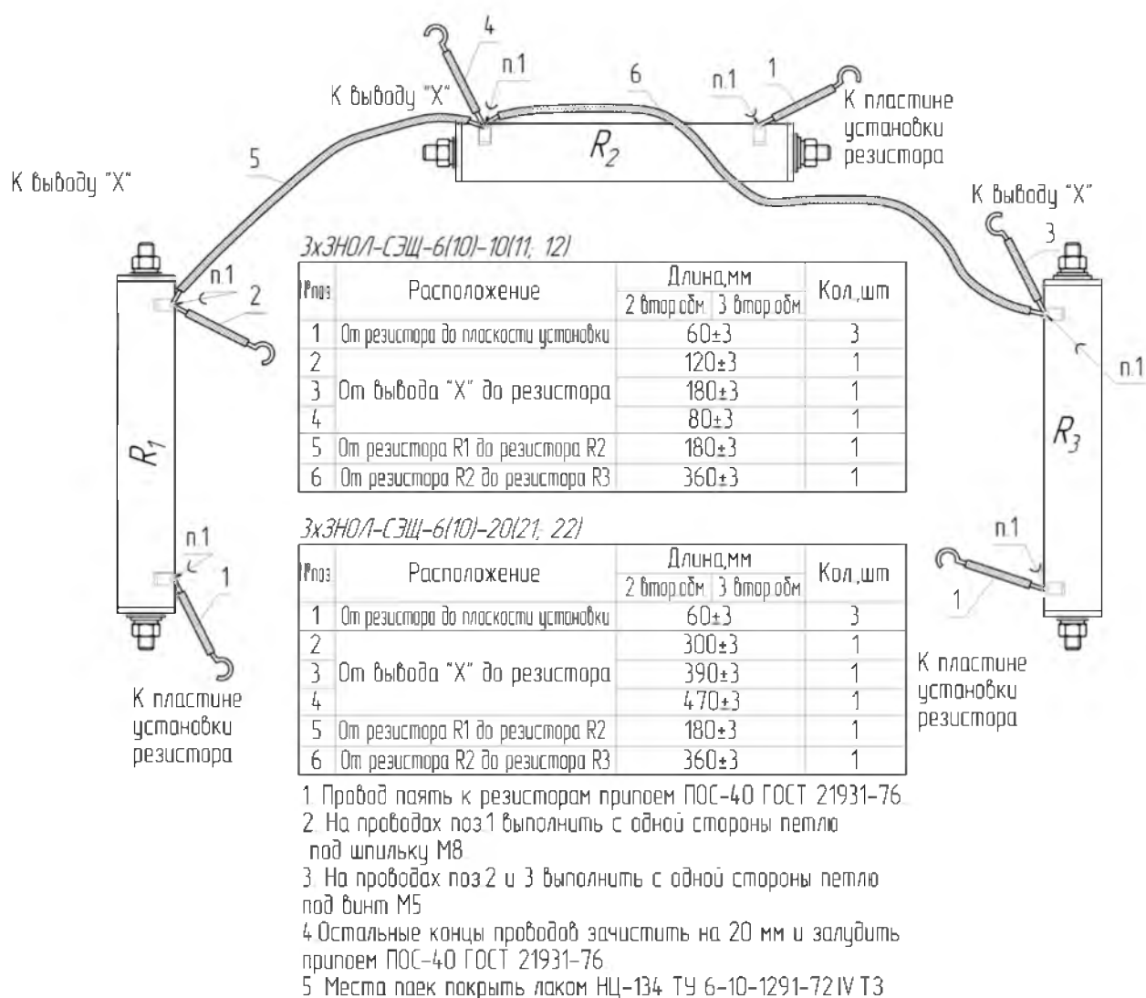
Рис.В.4 Монтажная схема соединения резисторов для трансформаторов 3хЗНОЛ-СЭЩ-6(10)-10(11; 12) и 3хЗНОЛ-СЭЩ-6(10)-20(21; 22)
