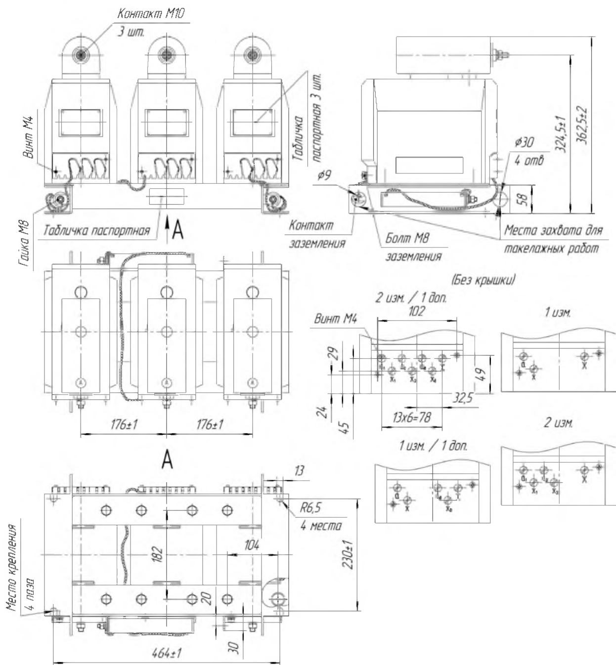
Рис.А.7 Габаритные, установочные и присоединительные размеры трехфазной группы измерительных трансформаторов
