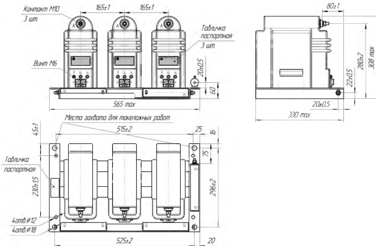
Рис.А.11 Габаритные, установочные и присоединительные размеры трехфазной группы измерительных трансформаторов
