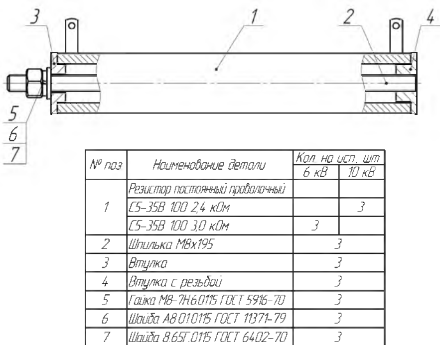
Рис.В.2 Сборка резисторов 3хЗНОЛ-СЭЦ-6(10)-10(20; 11; 12; 21; 22; 11М; 12М; 21М; 22М)
