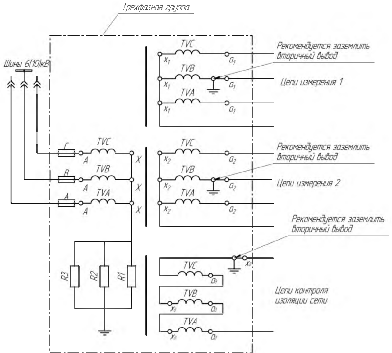
Рис.Б.8 Принципиальная электрическая схема соединения обмоток трехфазной группы измерительных трансформаторов 3 x ЗНОЛ – СЭЦ – 6(10) – 11(12; 21; 22) с тремя вторичными обмотками
