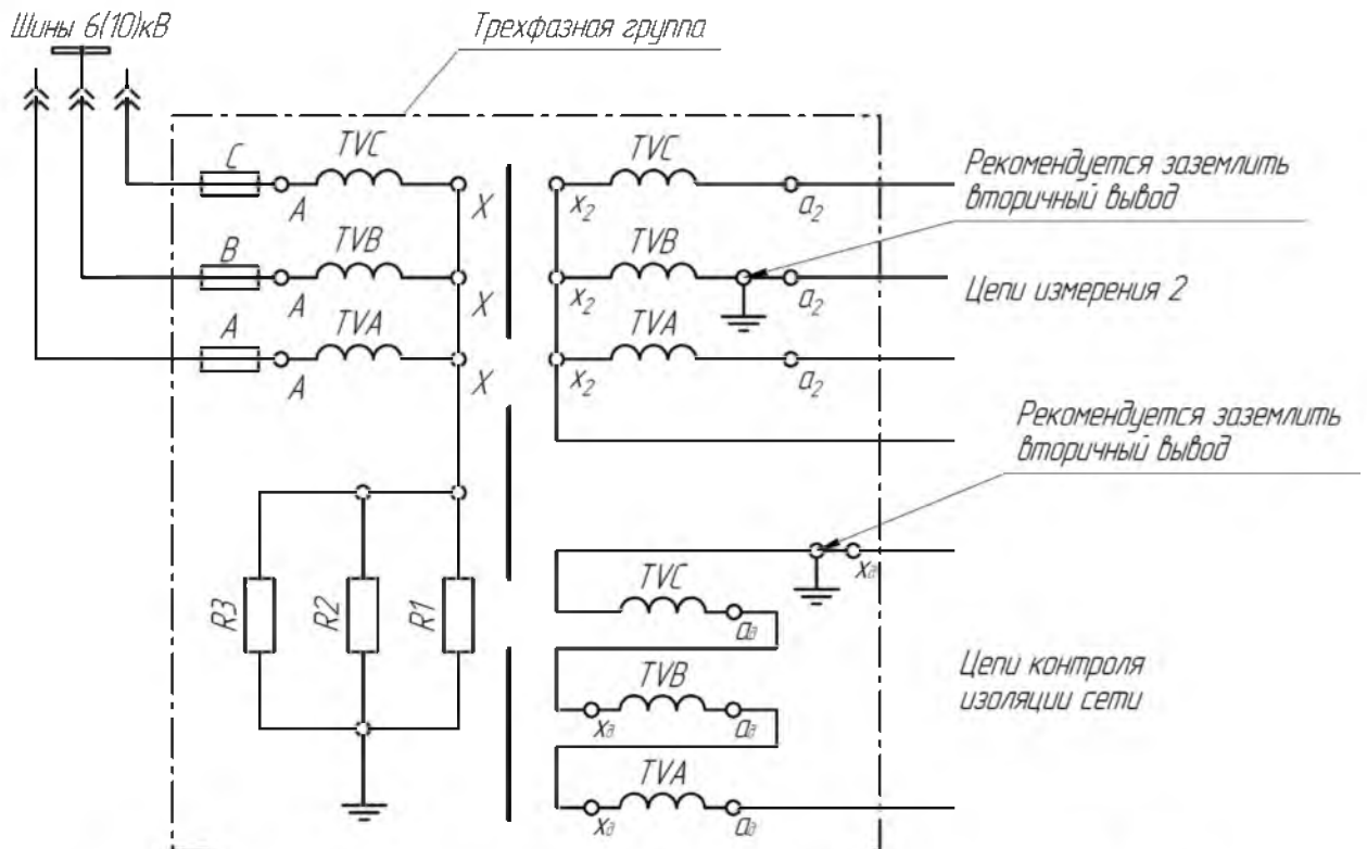
Рис.Б.4 Принципиальная электрическая схема соединения обмоток трехфазной группы измерительных трансформаторов 3 х ЗНОЛ – СЭЩ – 6(10) – 11(12; 21; 22)
