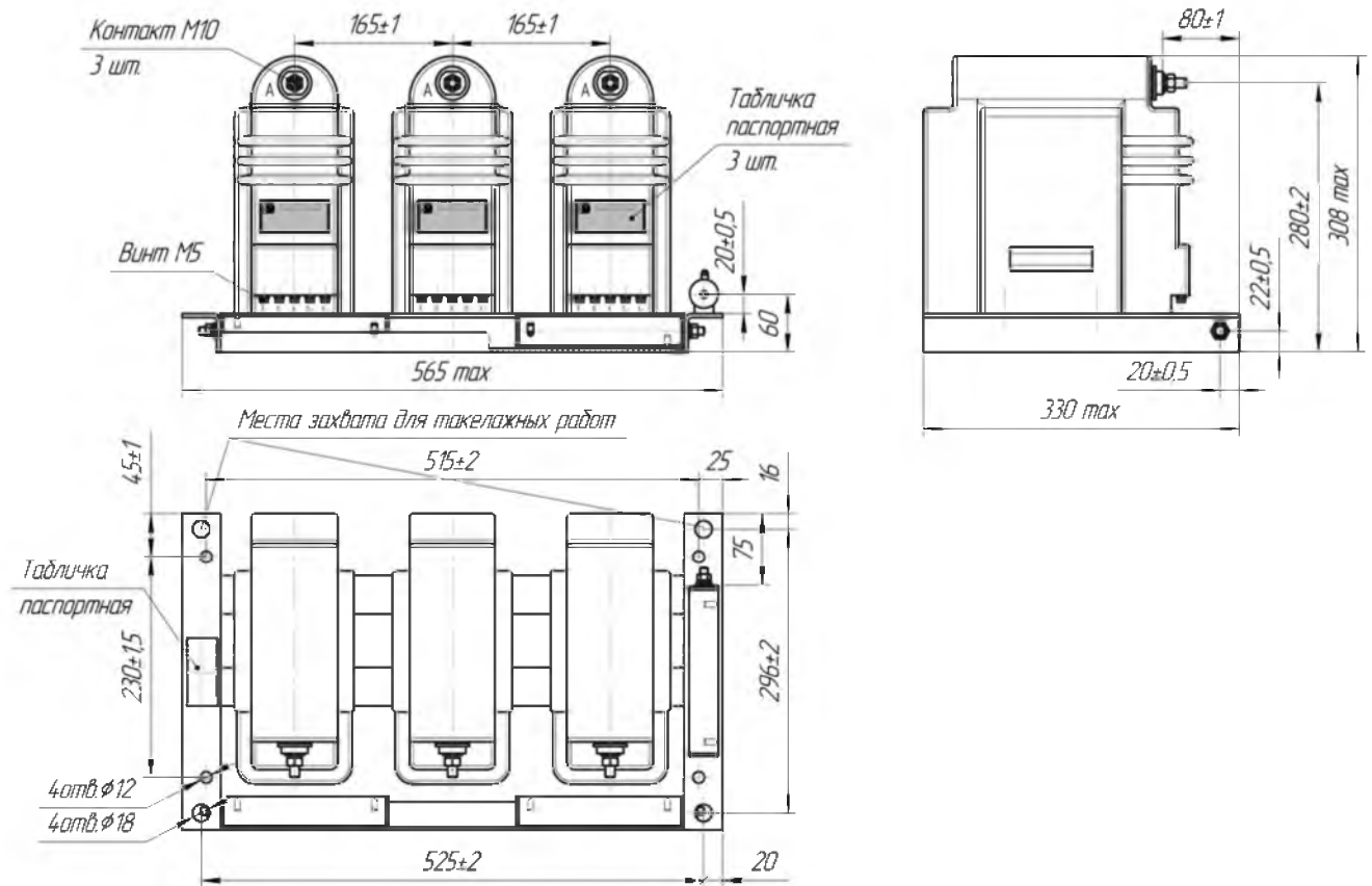
Рис.А.9 Габаритные, установочные и присоединительные размеры трехфазной группы измерительных трансформаторов 3 x ЗНОЛ – СЭЦ – 6(10) – 11М
