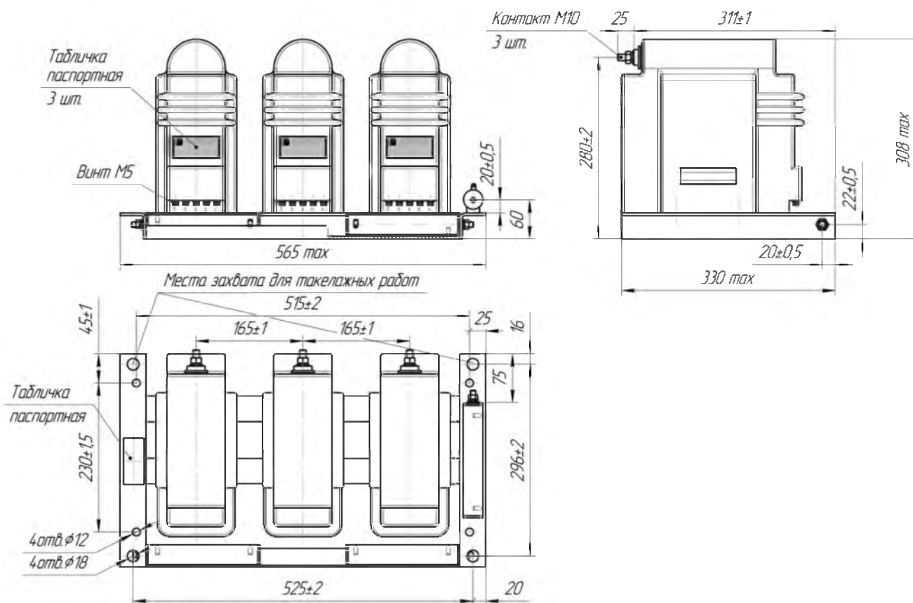
Рис.А.10 Габаритные, установочные и присоединительные размеры трехфазной группы измерительных трансформаторов
