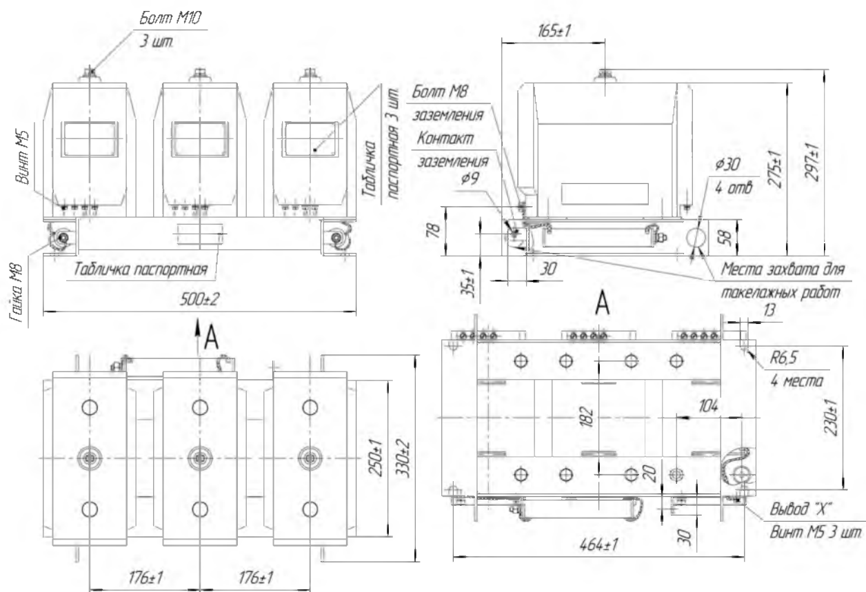
Рис.А.2 Габаритные, установочные и присоединительные размеры трехфазной группы измерительных трансформаторов
