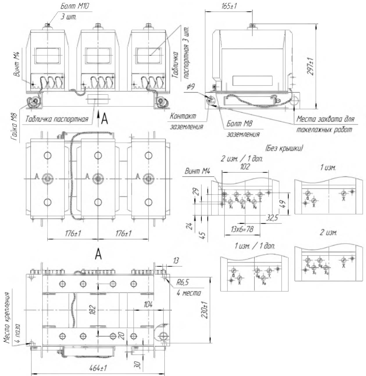
Рис.А.3 Габаритные, установочные и присоединительные размеры трехфазной группы измерительных трансформаторов 3 x ЗНОЛ – СЭЦ – 6(10) – 20
