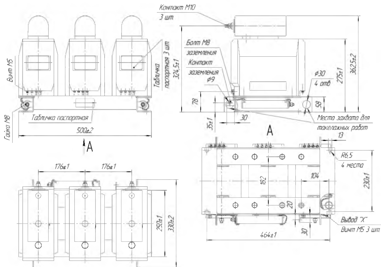
Рис.А.6 Габаритные, установочные и присоединительные размеры трехфазной группы измерительных трансформаторов 3 x ЗНОЛ – СЭЩ – 6(10) – 12
