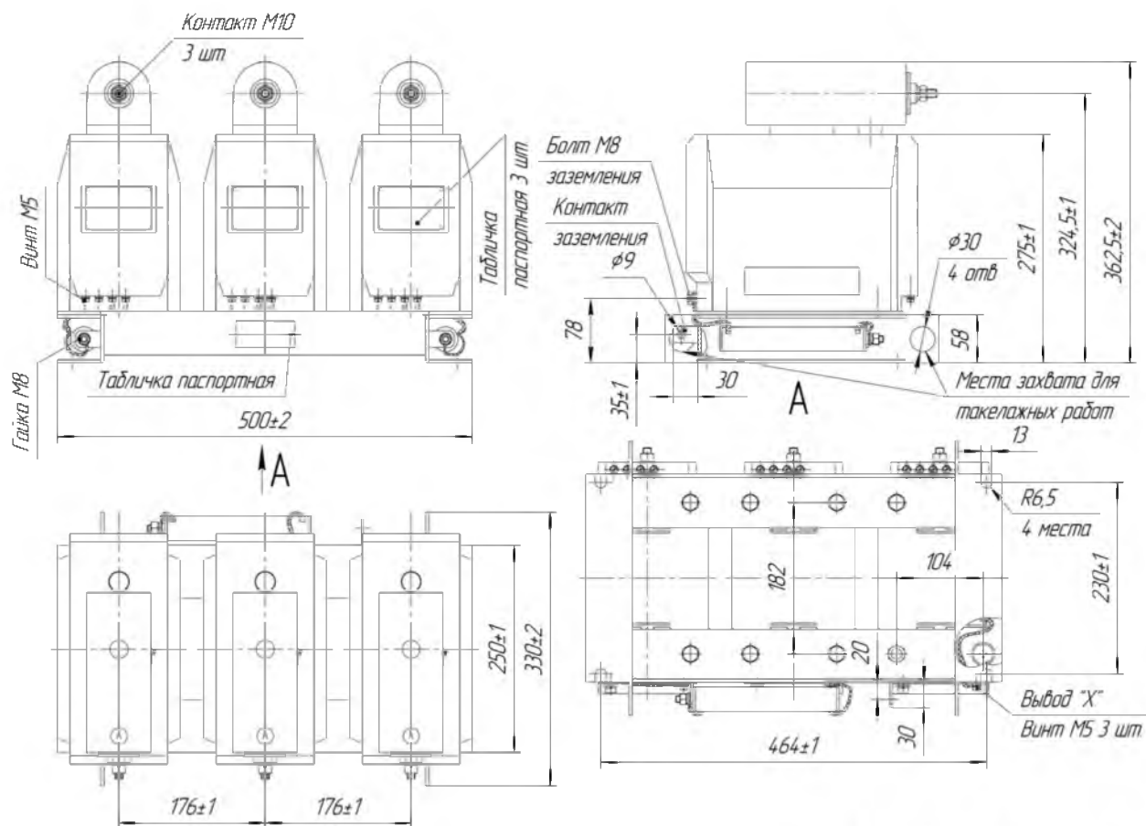
Рис.А.5 Габаритные, установочные и присоединительные размеры трехфазной группы измерительных трансформаторов
