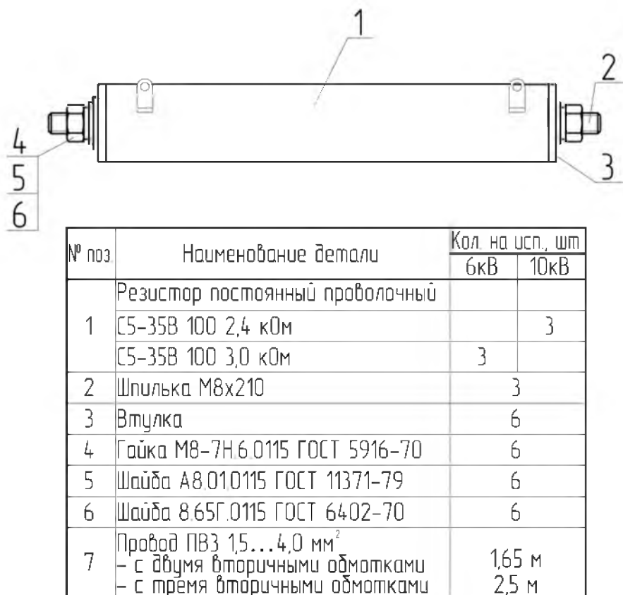
Рис.В.1 Сборка резисторов 3хЗНОЛ-СЭЦ-6(10)-(1)
